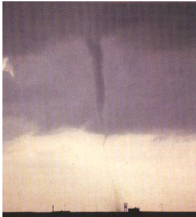
Figura 66 – Tornado
